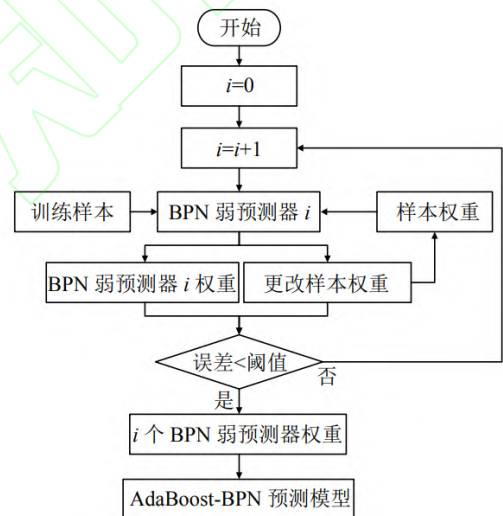
图 2 AdaBoost-BP 网络模型流程图 [18]
