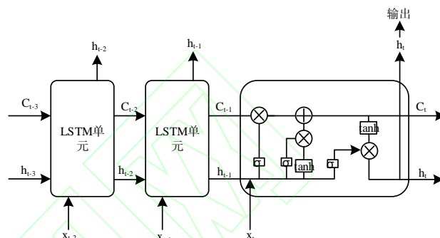
图9 LSTM结构示意图 Fig.9 Schematic of LSTM structure
