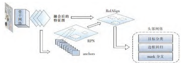
图 3 Mask R-CNN 模型图 [30]
