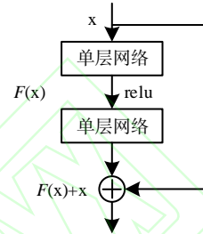
图 7 ResNet 跳跃连接
