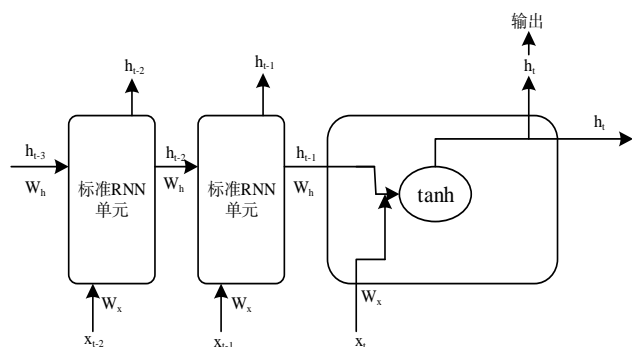
图8 RNN结构示意图 Fig.8 Schematic of RNN structure
