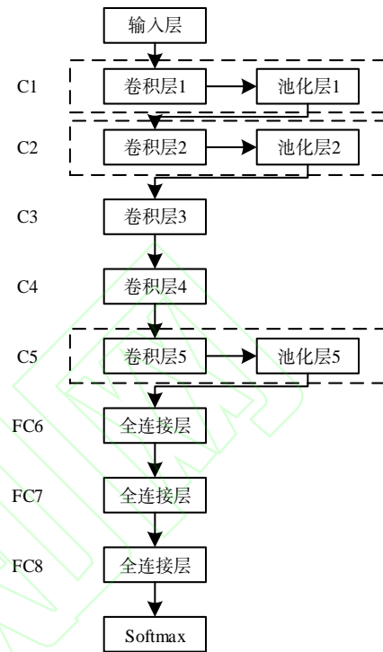
图 4 AlexNet 示意图
