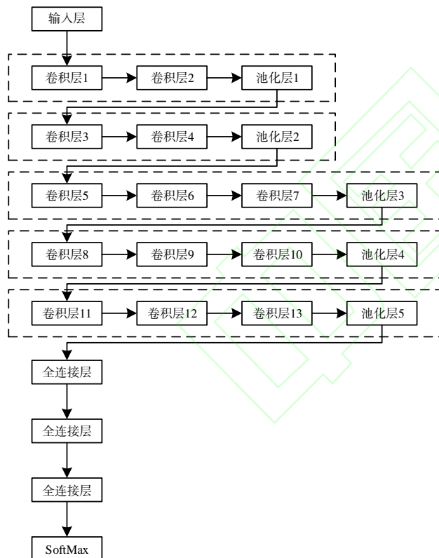
图 5 VGG-16 示意图
