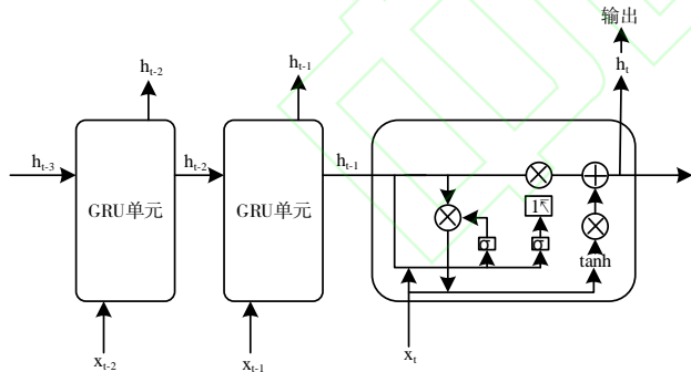
图 10 GRU 结构示意图
