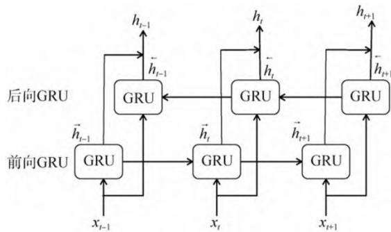
图 11 BiGRU 结构示意图 [91]
