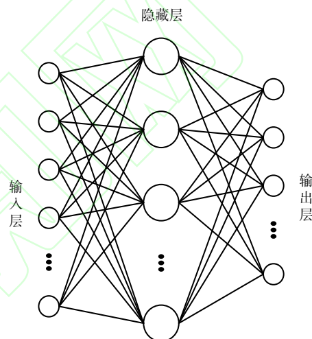
图 1 MLP 结构示意图
